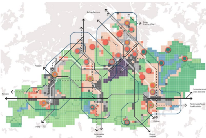
Leitbild Flughafenregion Airport Berlin-Brandenburg
